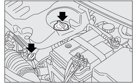
fig. 9 - versioni 1.6 Multijet
